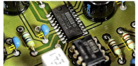
Doskonale, chociaż od dawna nieprodukowane układy – przetworniki C/A Burr Brown PCM1704 w selekcjonowanej wersji „K”.
