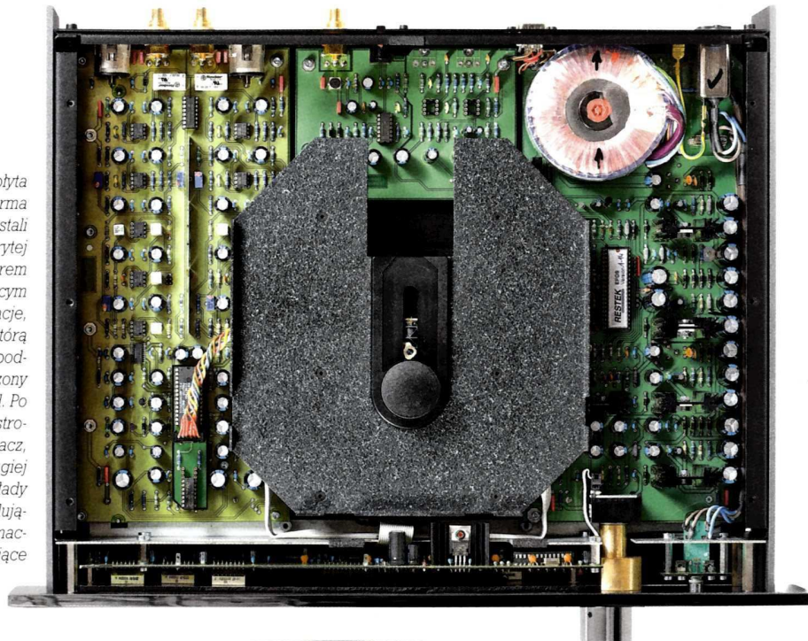
Doskonale, chociaż od dawna nieprodukowane układy – przetworniki C/A Burr Brown PCM1704 w selekcjonowanej wersji „K”.
